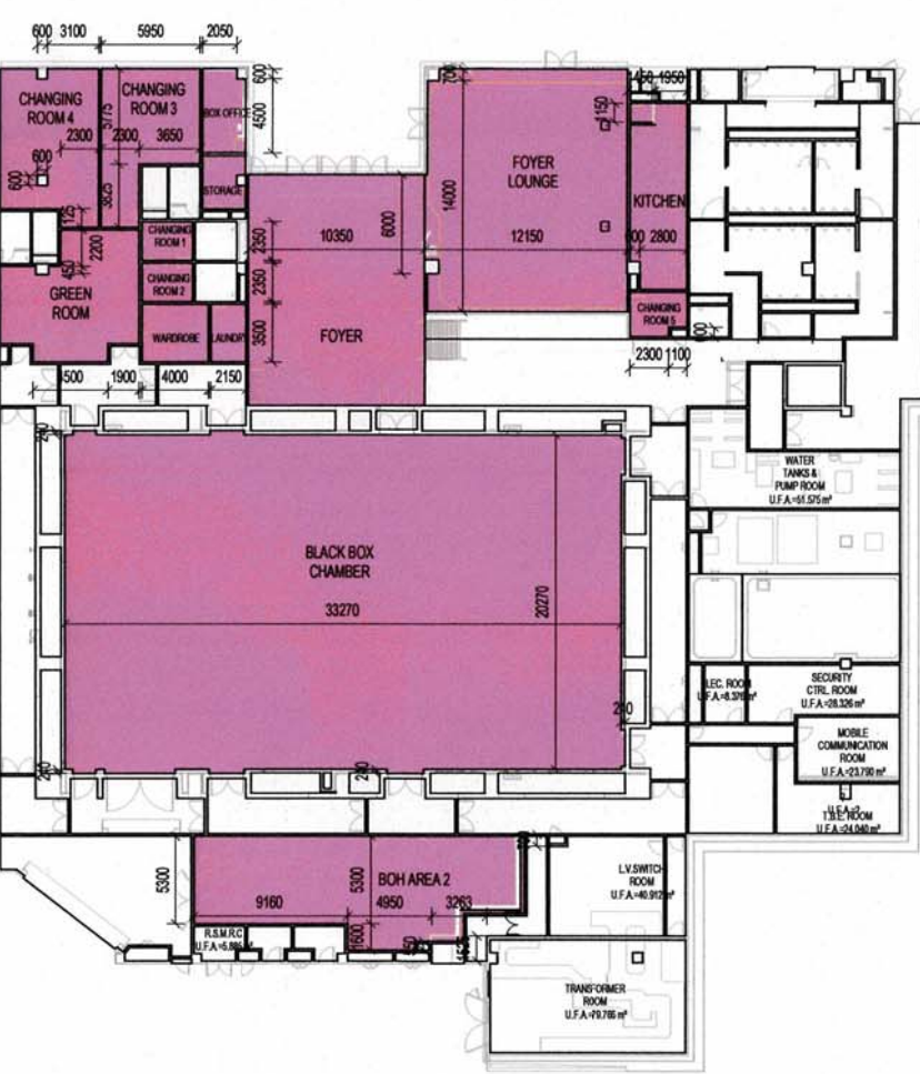
G/F U.F.A. DIAGRAM
