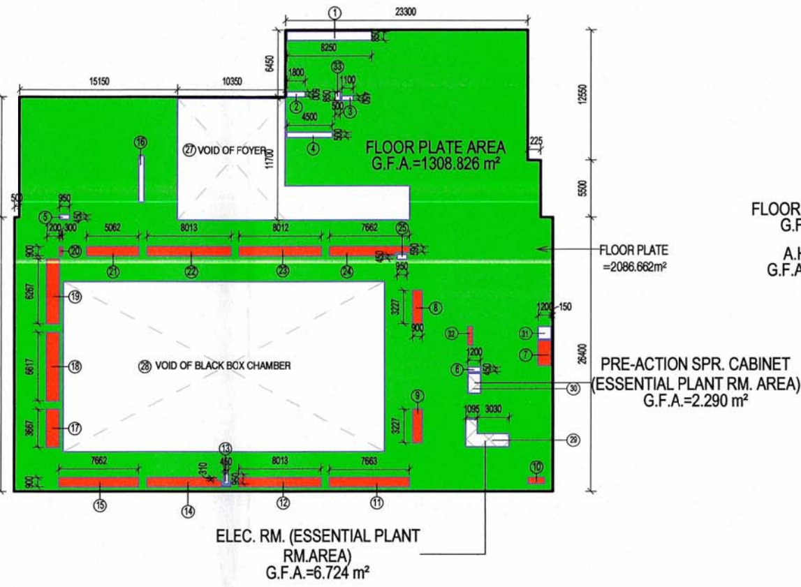
1/F G.F.A. DIAGRAM
